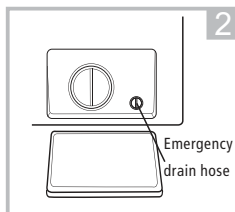
2 Virar 90° e retirar a mangueira de drenagem de emergência e retirar a tampa da mangueira.
